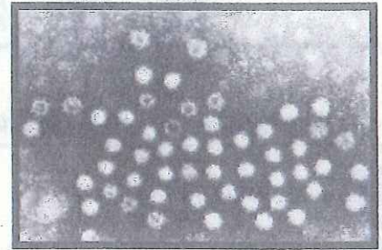
ノロウイルスの電子顕微鏡写真
